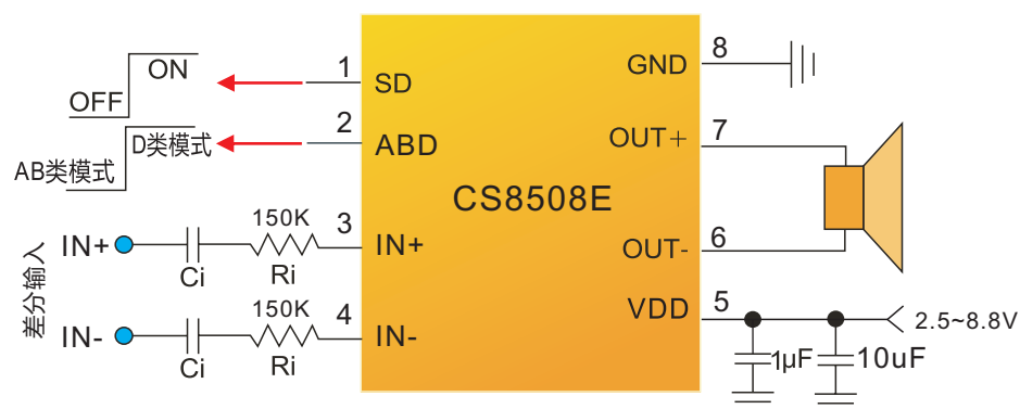
CS8508E应用电路图
